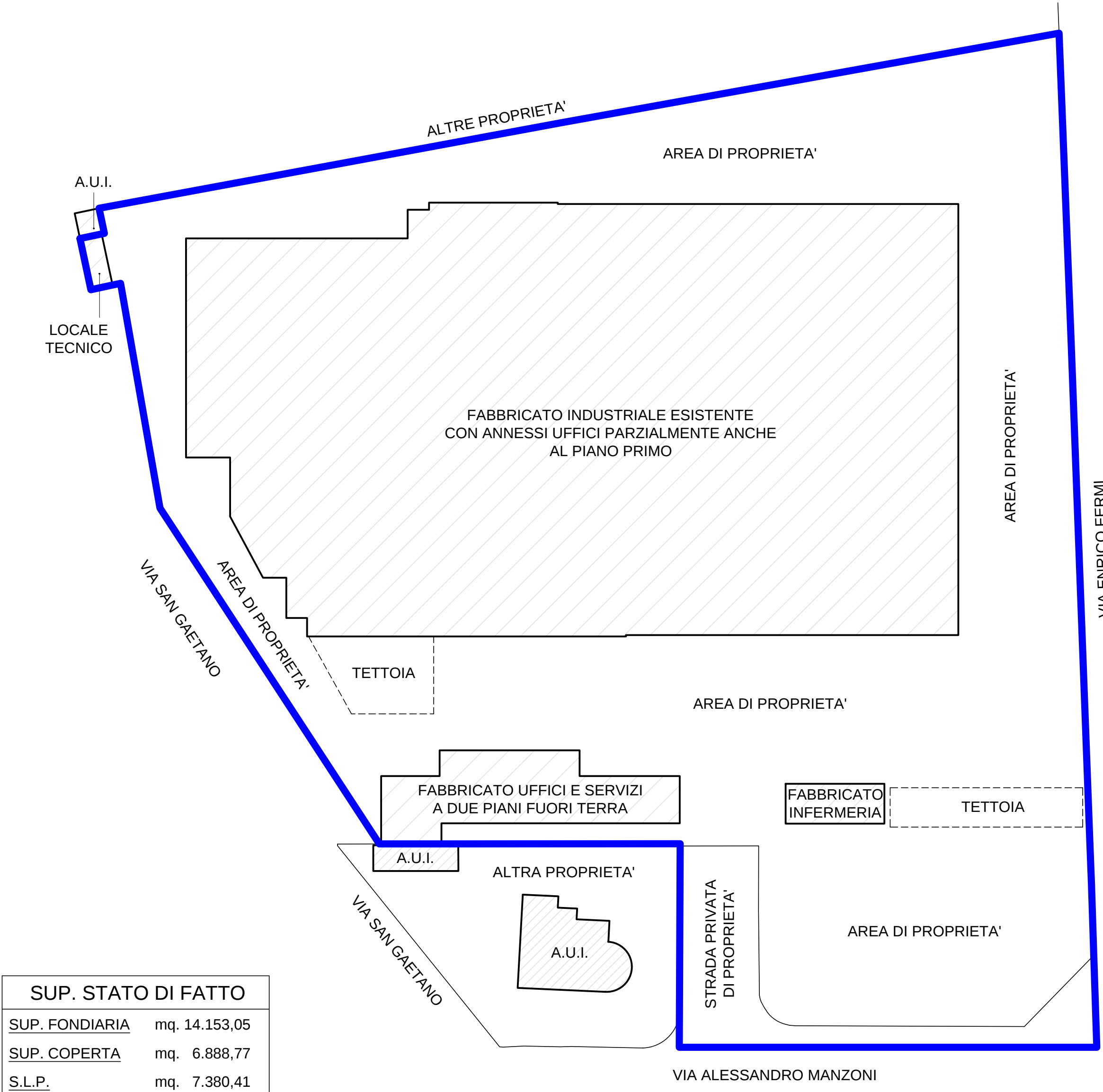
PLANIMETRIA GENERALE E PIANTA PIANO TERRA (stato di fatto)
