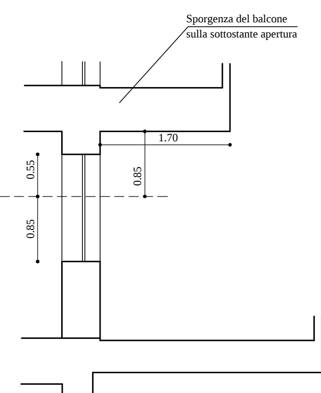
PARTICOLARE FINESTRA BAGNI APPARTAMENTI 5 e 6
