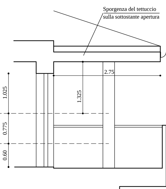
PARTICOLARE PORTA FINESTRA CUCINA APPARTAMENTO 4
