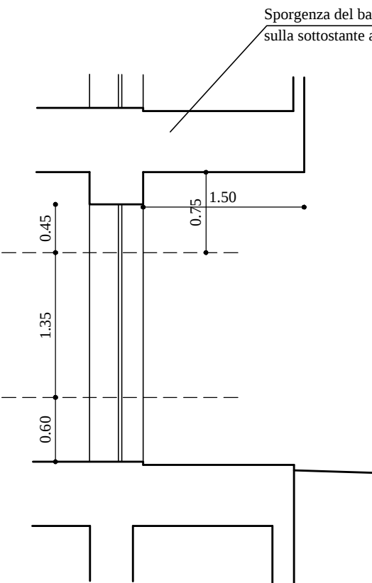
PARTICOLARE PORTA FINESTRA CUCINA APPARTAMENTO 7 E 9
