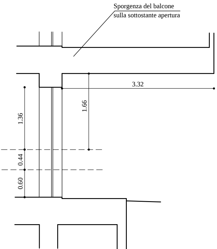
PARTICOLARE PORTA FINESTRA SOGGIORNO APPARTAMENTO 9
