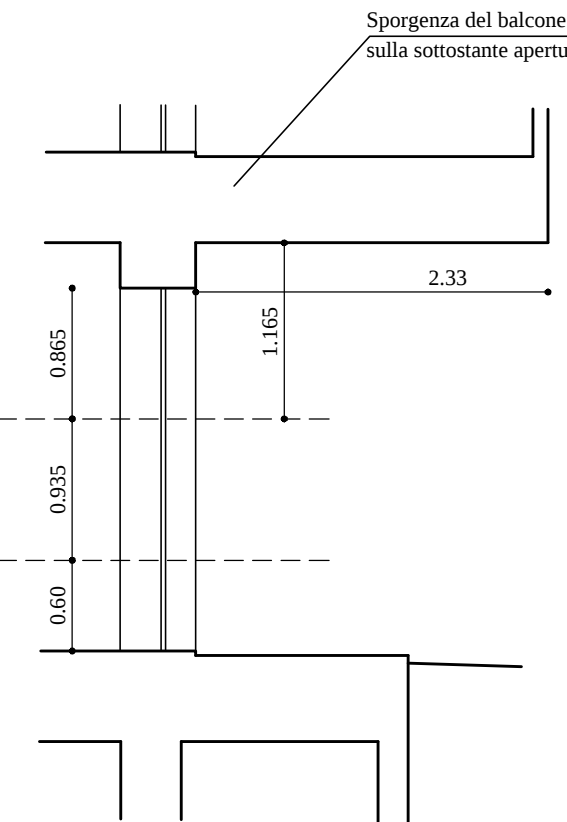
PARTICOLARE PORTA FINESTRA CUCINA APPARTAMENTO 3
