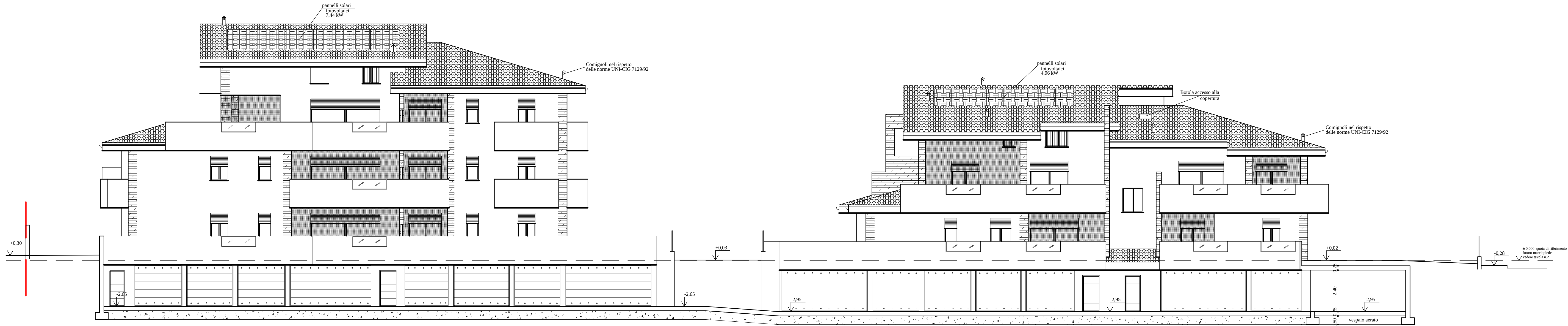
SEZIONE E-E PROSPETTO OVEST
