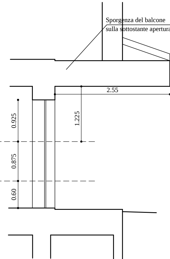
PARTICOLARE PORTA FINESTRA SOGGIORNO APPARTAMENTO 1
