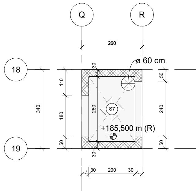
VISTA SPECULARE COPERTURA - CAMERETTA P02
