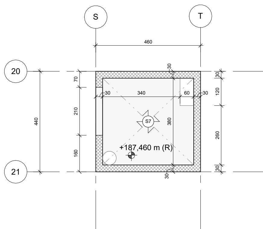
VISTA SPECULARE COPERTURA - CAMERETTA SF01
